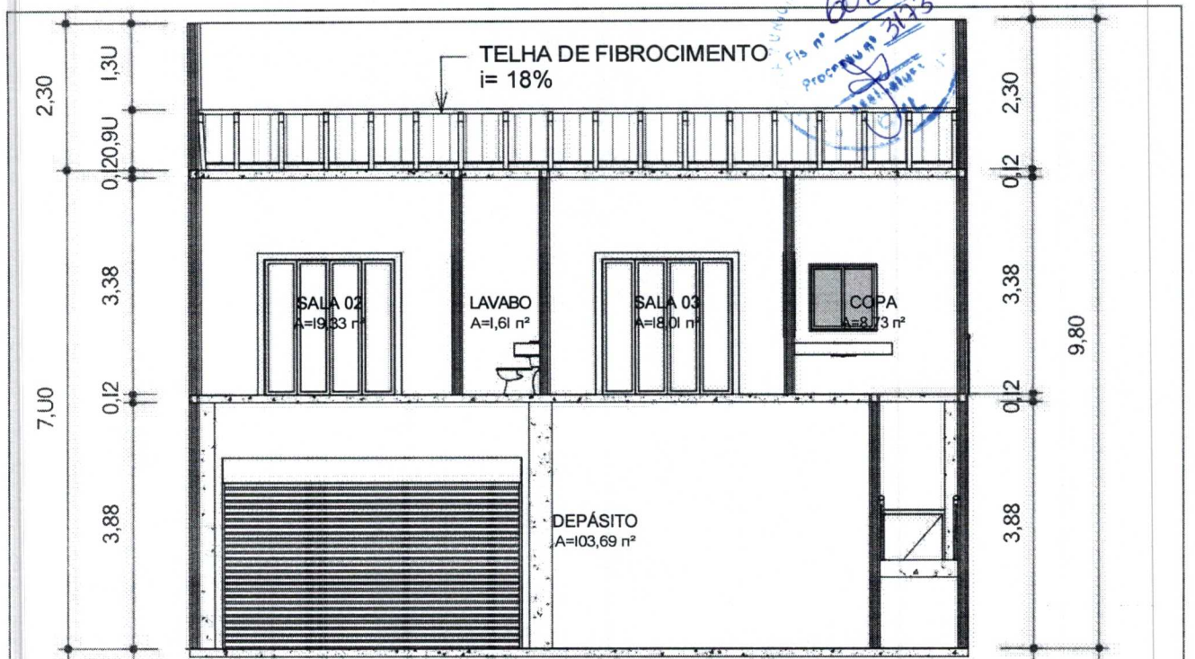
1 Corte 1 1 : 100
