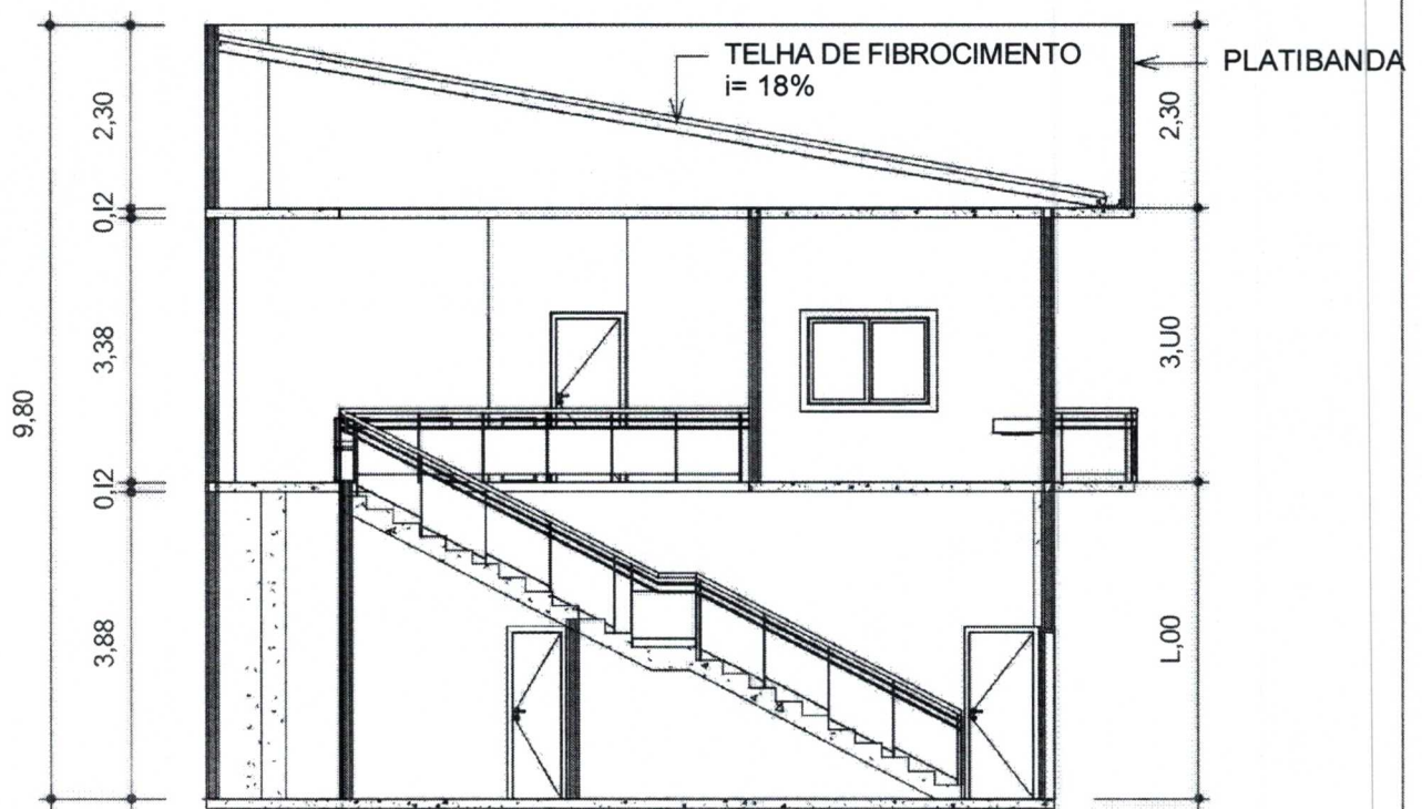
2 Corte 2 1 : 100
