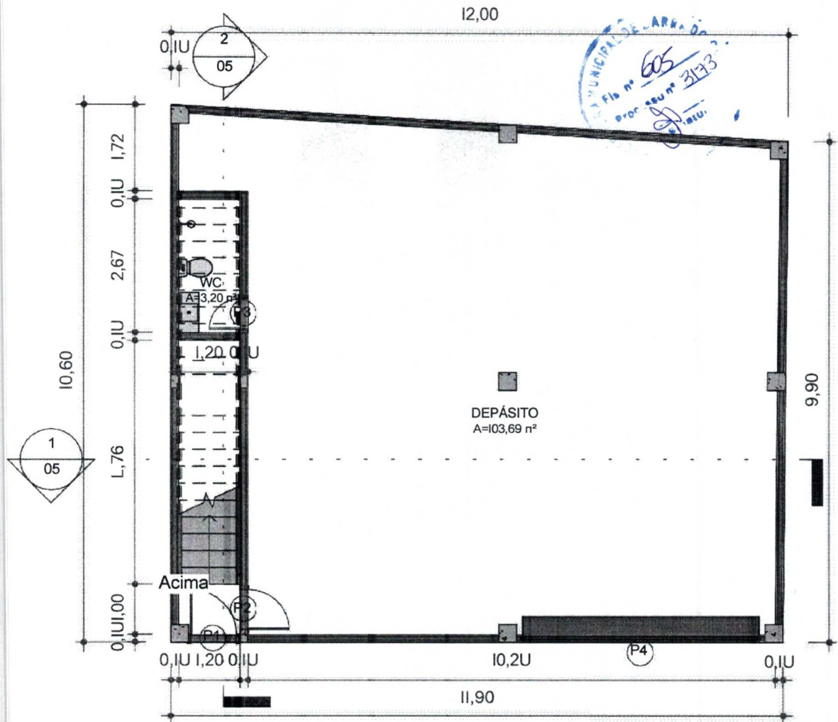
1 PLANTA BAIXA - TÉRREO 1 : 100
