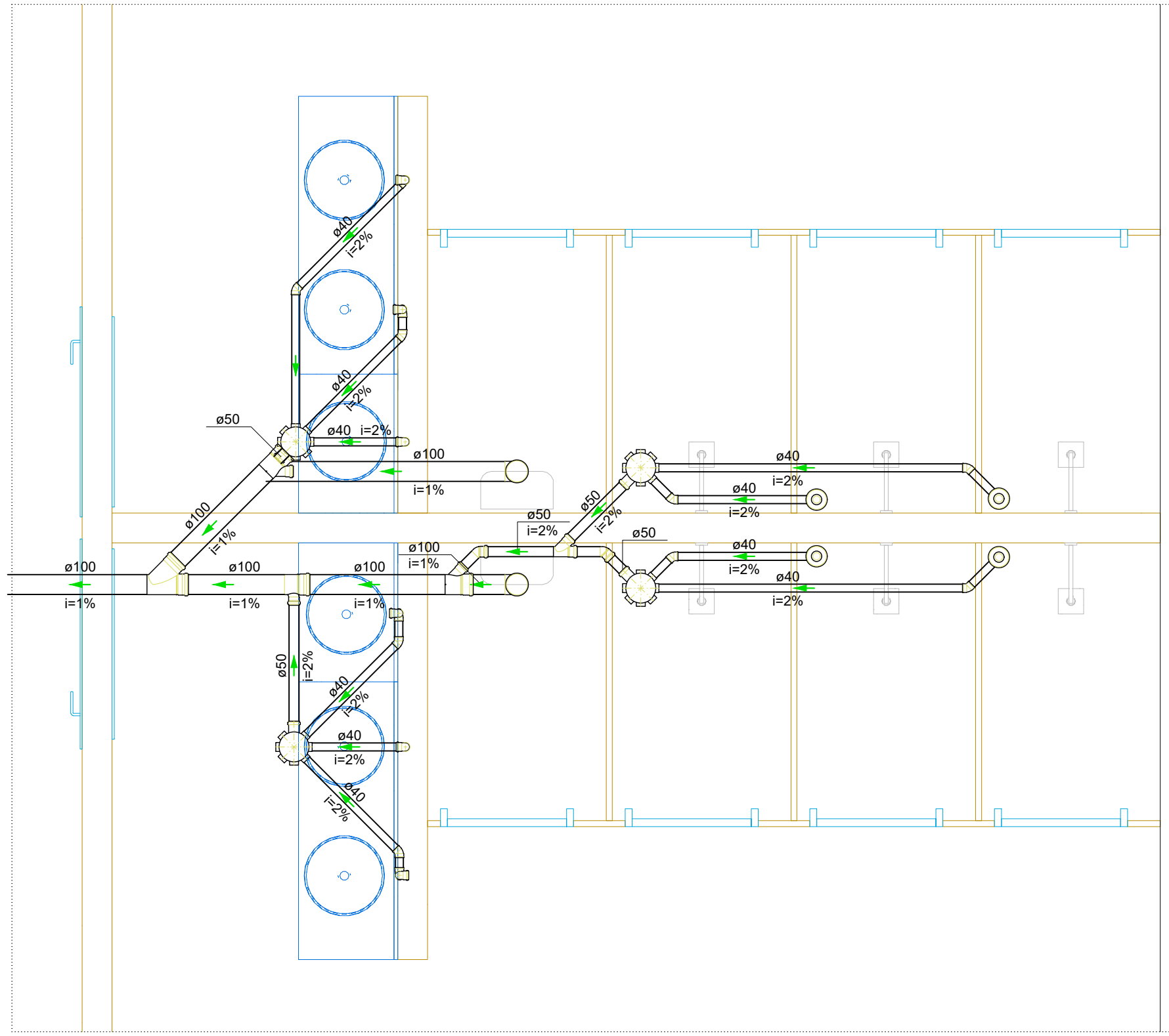
Detalhe SAN-7 Escala 1:25
