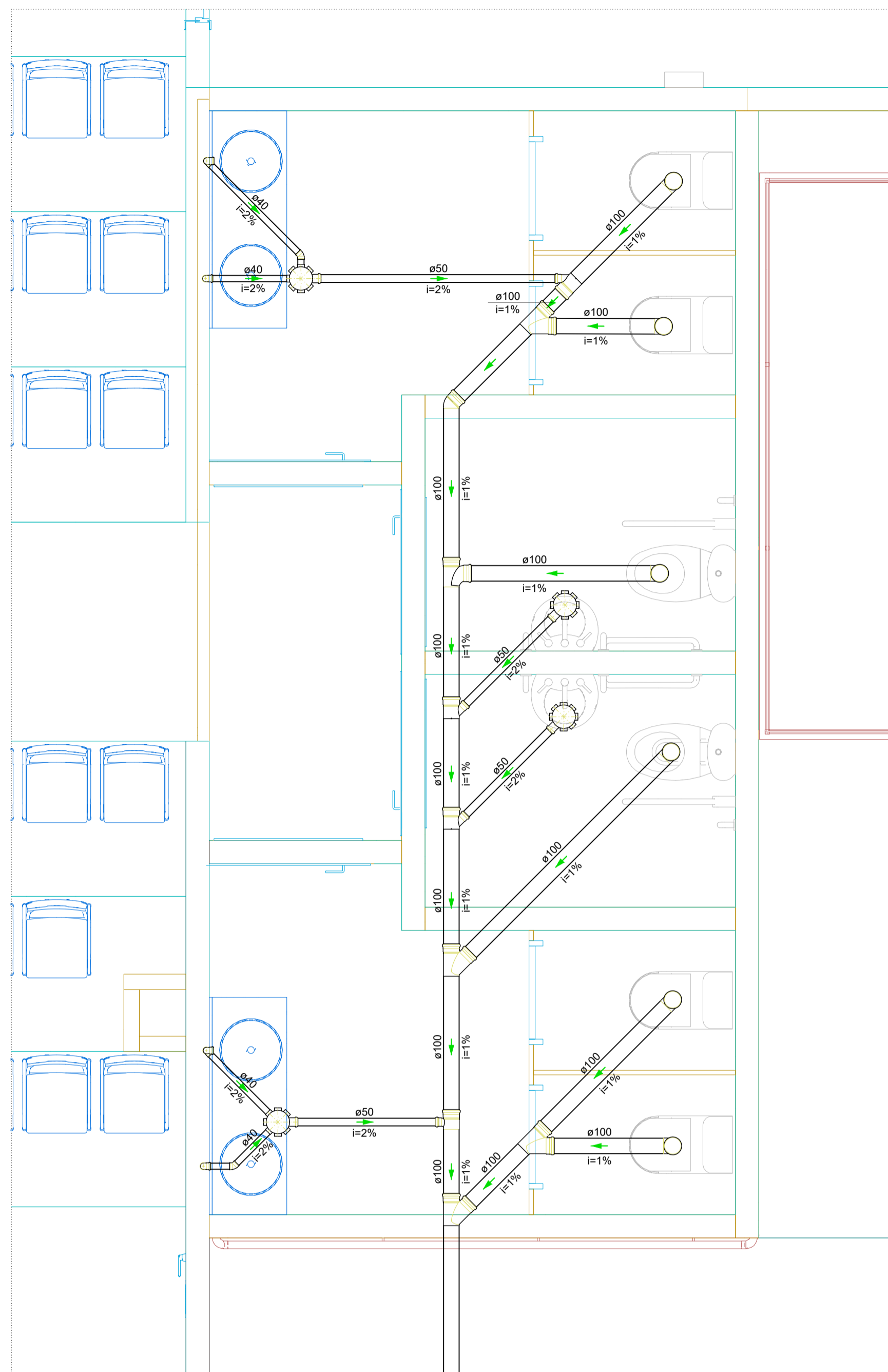
Detalhe SAN-3 Escala 1:25
