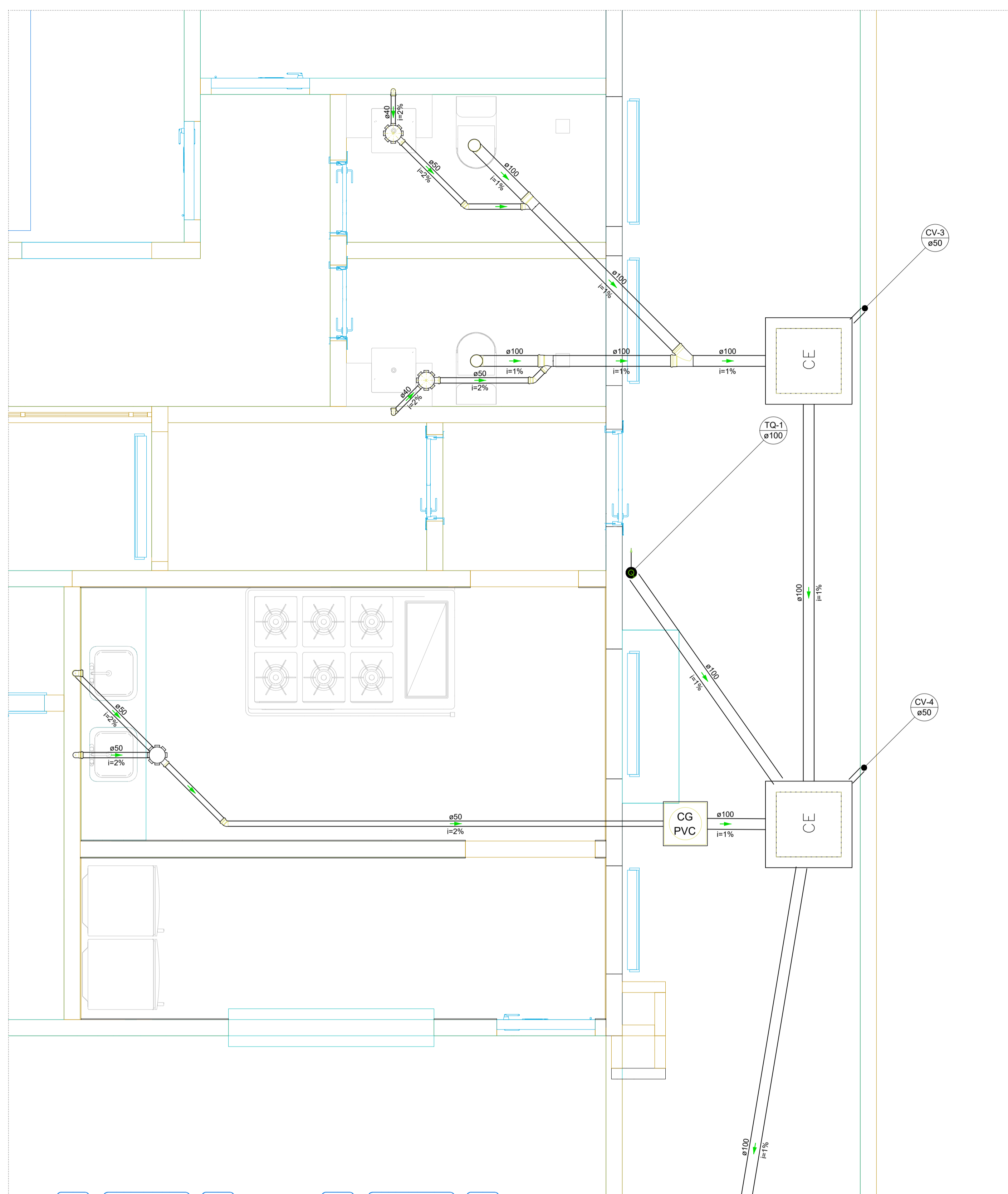
Detalhe SAN-4 Escala 1:25
