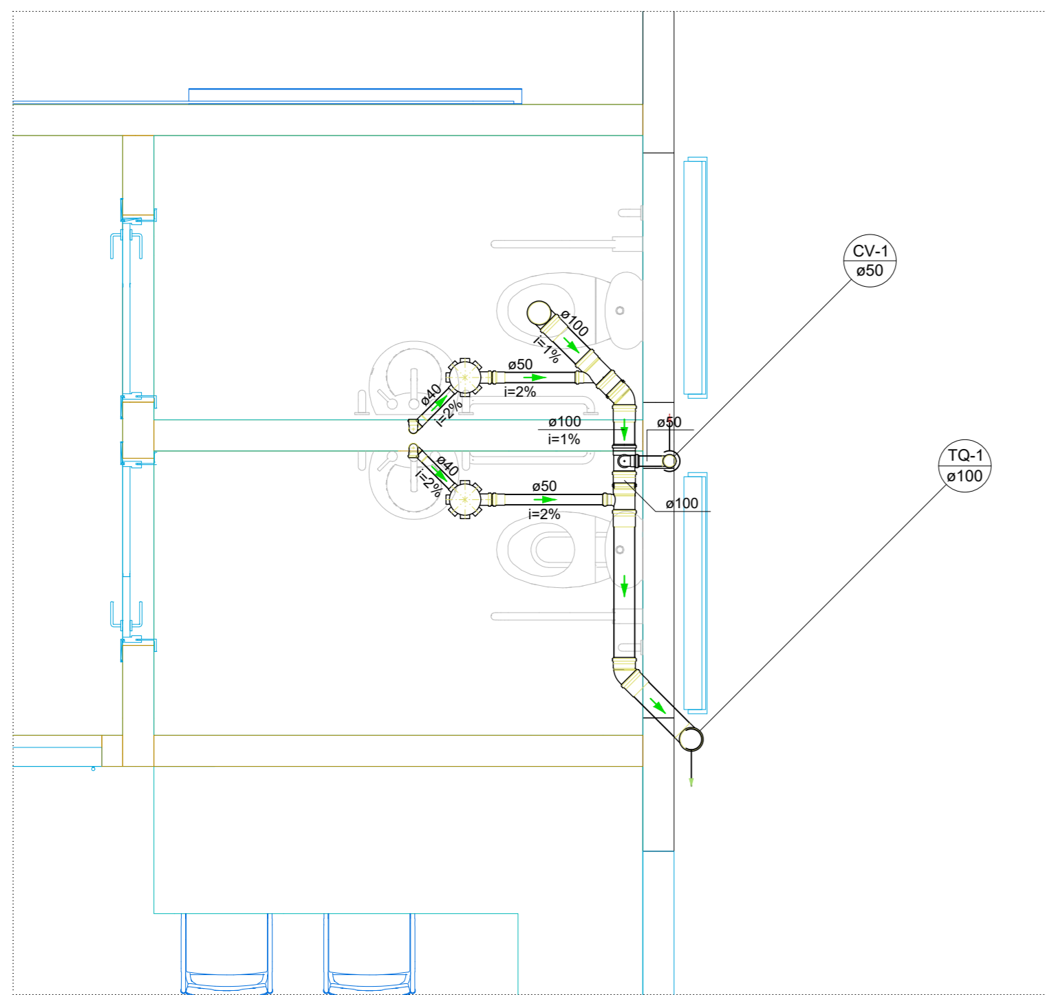
Detalhe SAN-1 Escala 1:25
