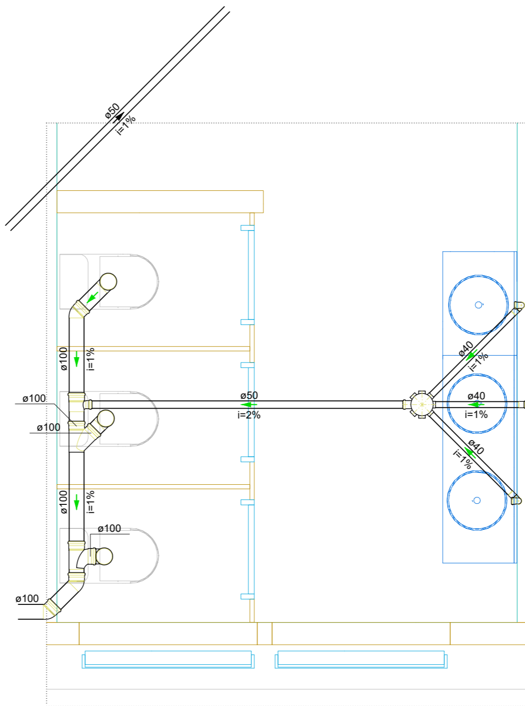
Detalhe SAN-2 Escala 1:25
