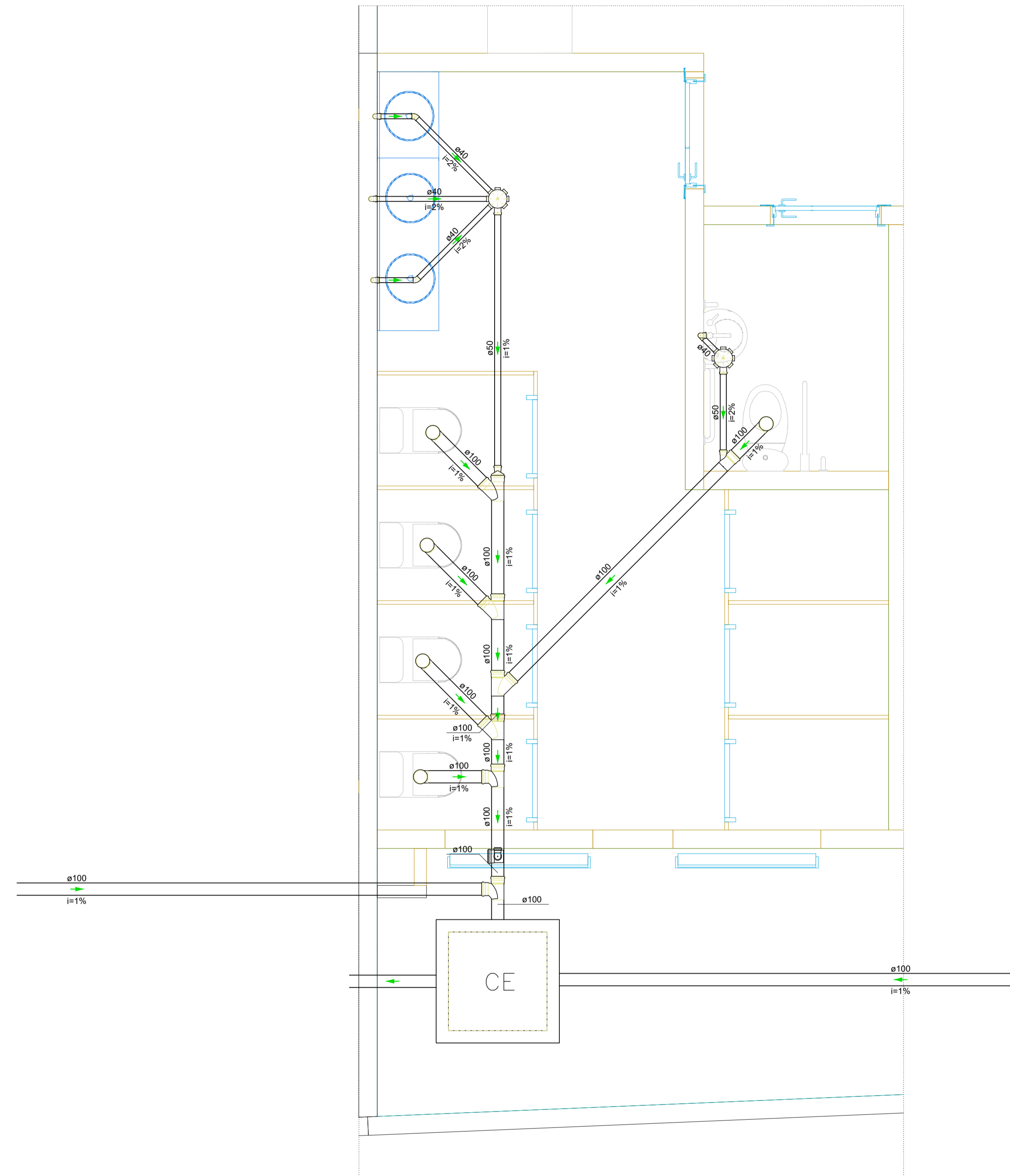
Detalhe SAN-6 Escala 1:25
