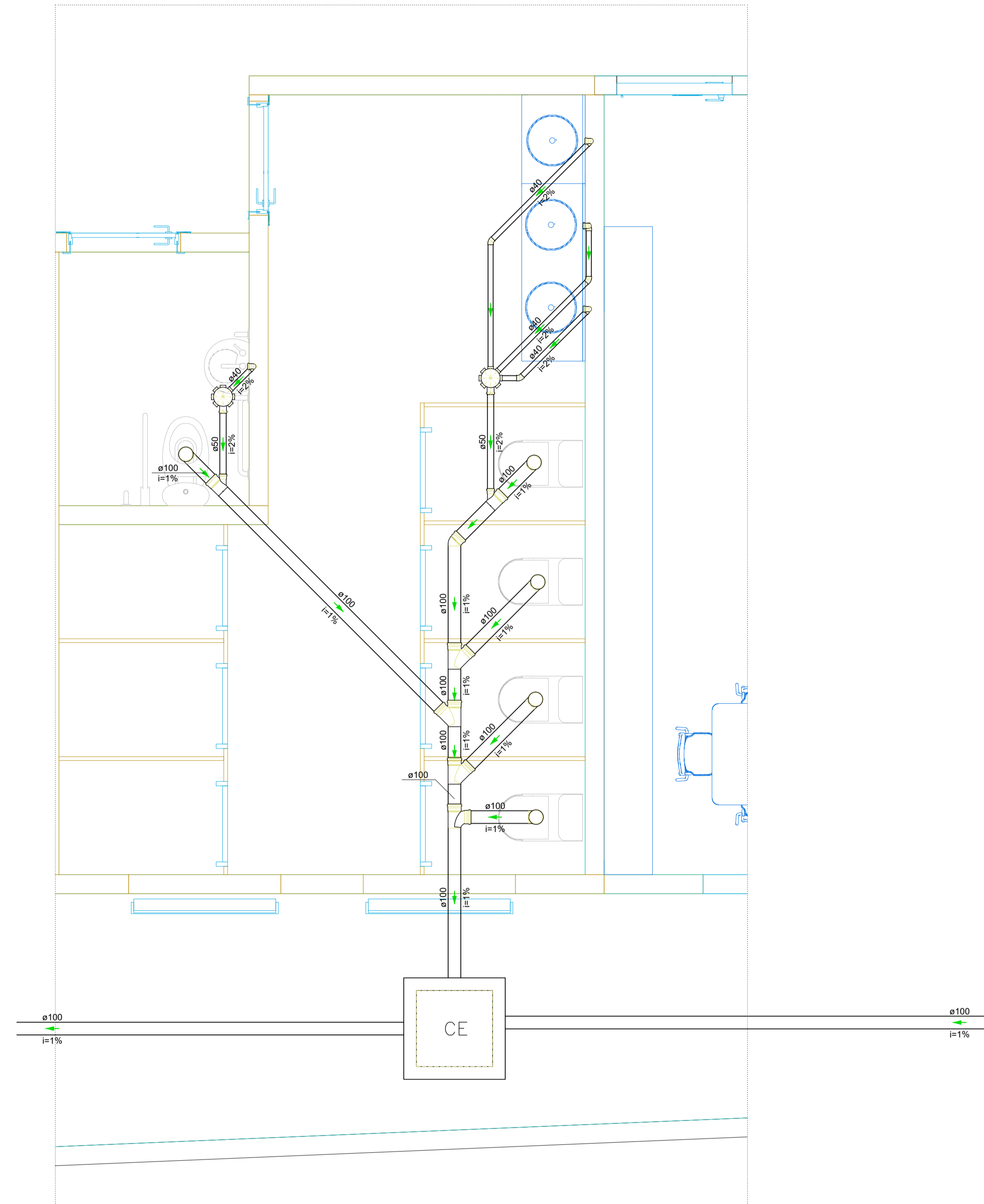
Detalhe SAN-5 Escala 1:25
